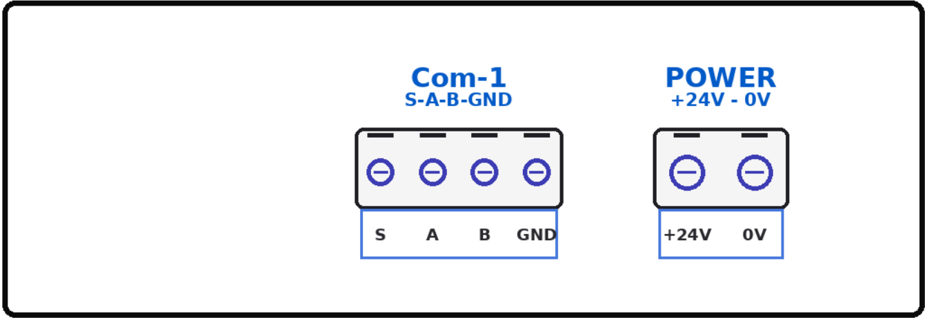
Şekil 1 – Modbus ve Güç Portu Yerleşimi
