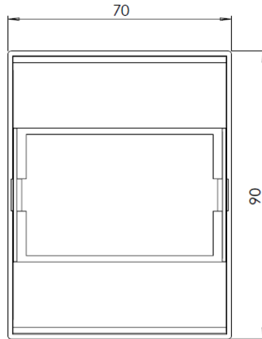
Şekil 2 – Dış kapak dahil kutu boyutları
