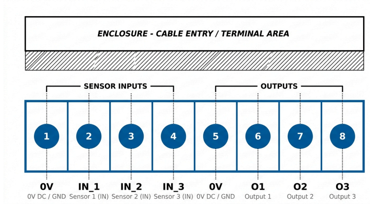
Şekil 1 – Bağlantı Şeması
