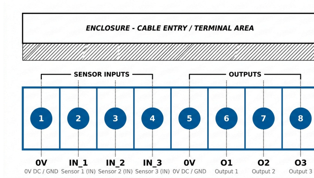
Şekil 4.1 - Bağlantı Şeması
